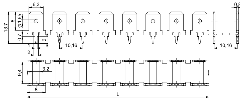
Masse im Steckbereich DIN46342, Teil 1
